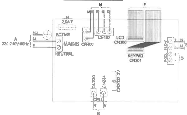
Anschlüsse Ei 2 Expert
